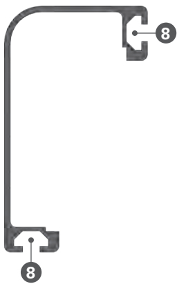
Profil Höhenverstellung
