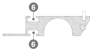
Funktionsprofil Toplight
